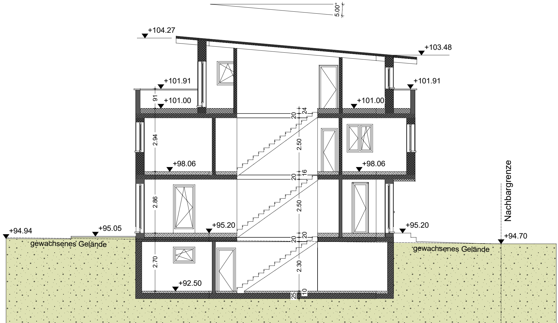
Schnitt A-A
