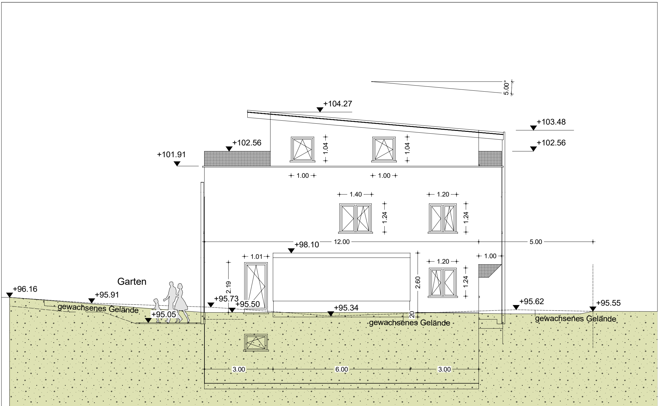
Ostansicht
