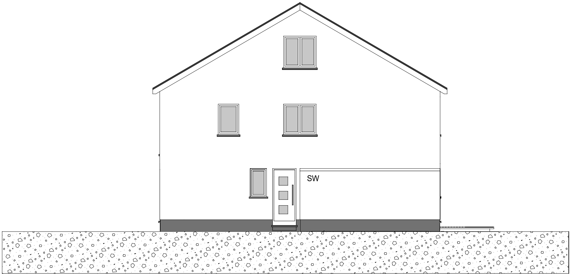
H04-07-Ansicht Giebelseite
