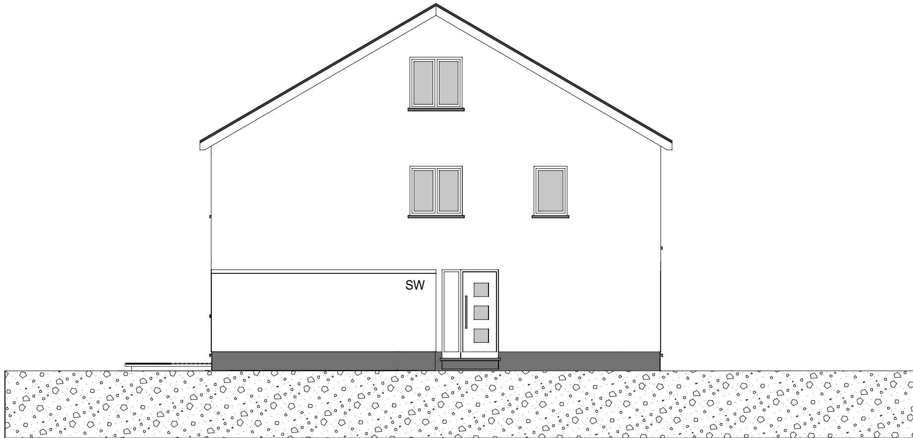
H04-05-Ansicht Giebelseite
