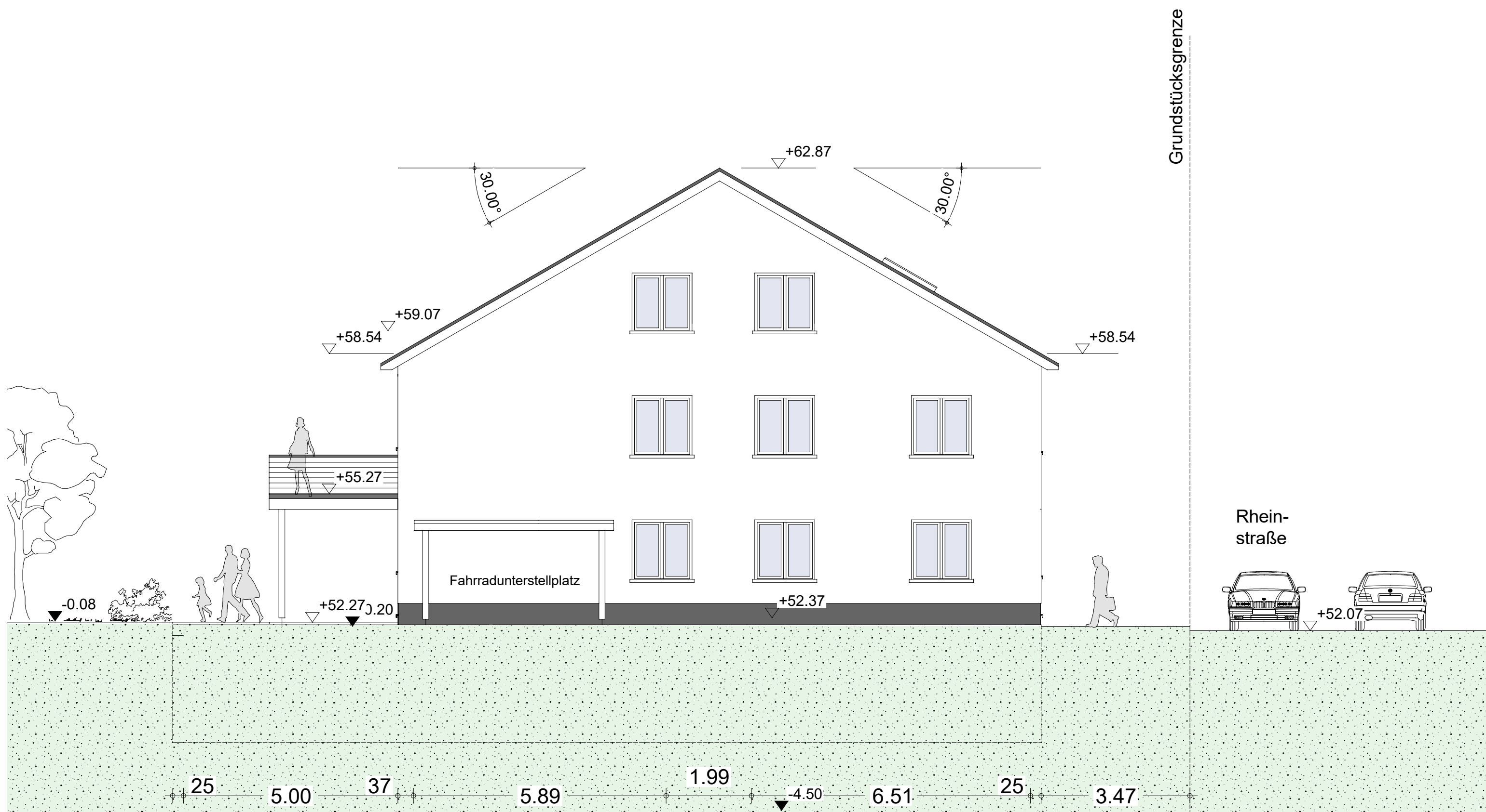
Ansicht-Süd
